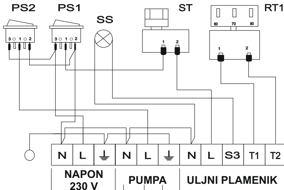
Slika 11. Električna shema kotlovske regulacije EKO-CK/CKB za ulje / plin i termostatske pumpe
