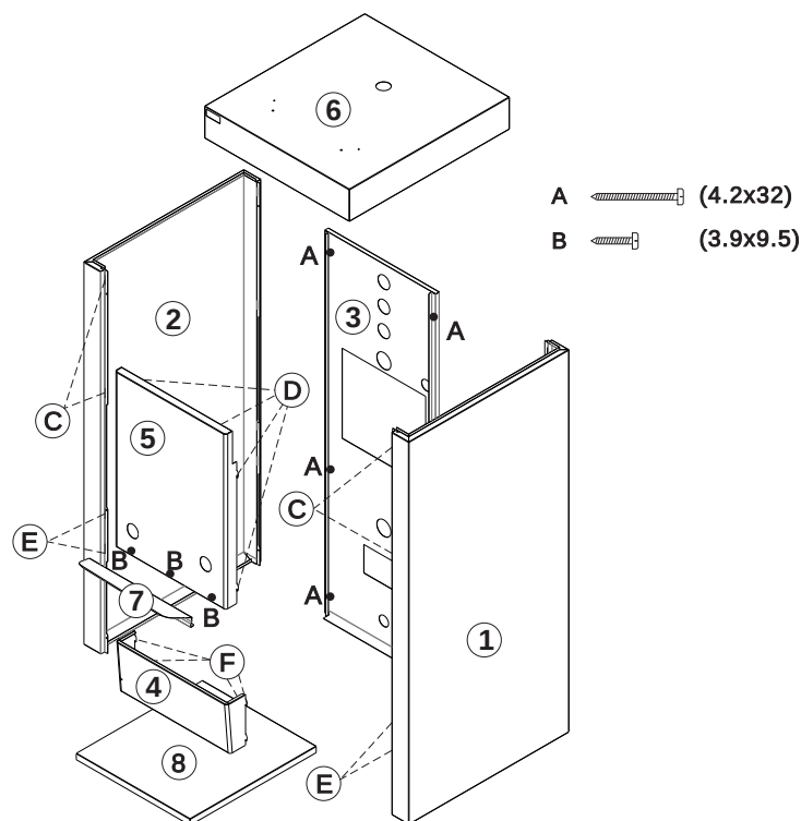
Slika 5. Postupak montaže oplave na kotao EKO-CKB P
