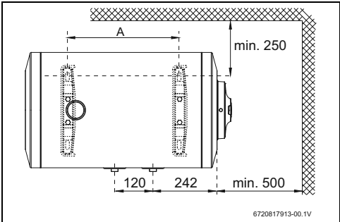
Sl.3 Dimenzije u mm (vodoravna montaža)
